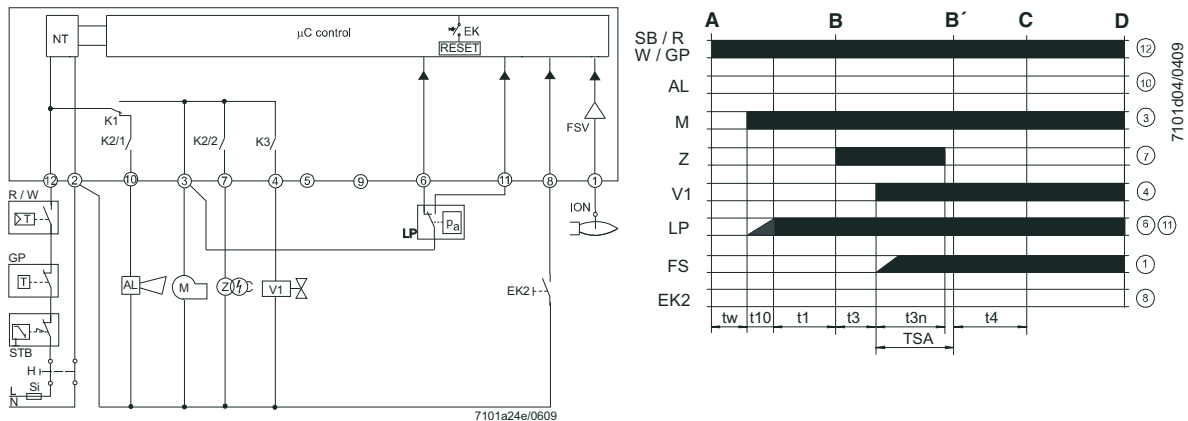
Diagrama de conexión y secuencia de control LME11...
