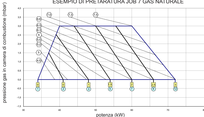
ESEMPIO DI PRETARATURA JOB 7 GAS NATURALE
