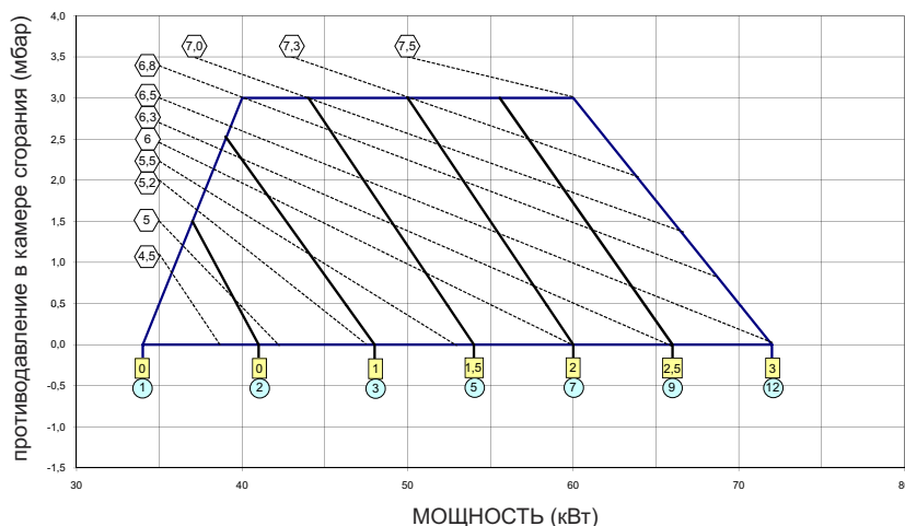
ПРИМЕР ПРЕДВАРИТЕЛЬНОЙ КАЛИБРОВКИ JOB 7
